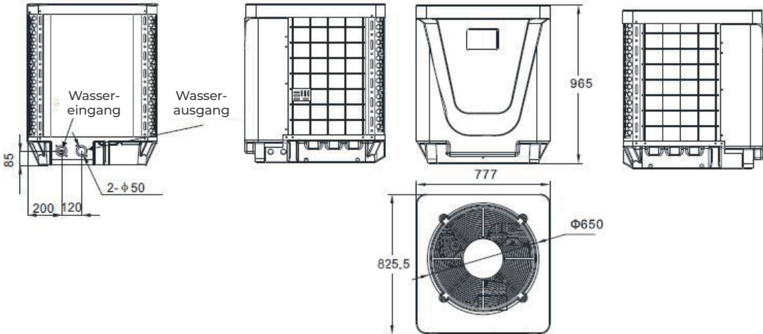
GERÄT: P31V/32/P31TV/32/P35V/32/P35TV/32 einheit mm
