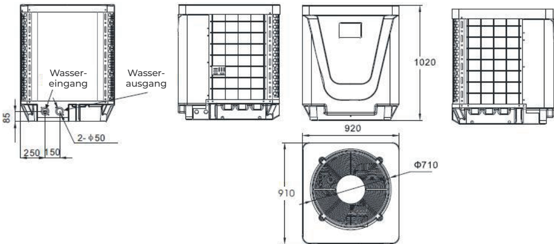
GERÄT: P31V/32/P31TV/32/P35V/32/P35TV/32 einheit mm
