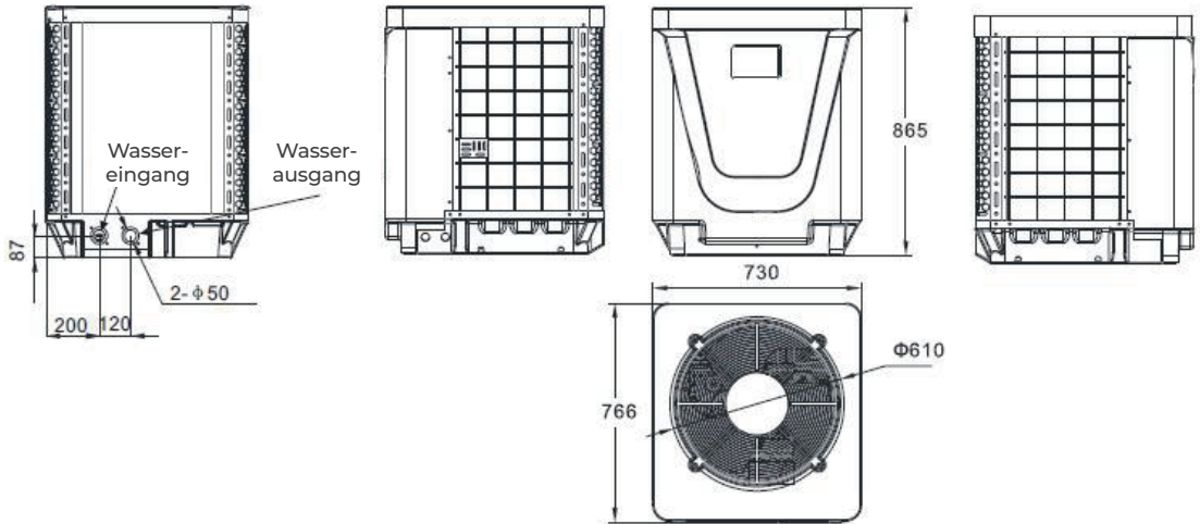
GERÄT: P21V/32/P21TV/32/P24V/32/P24TV/32 einheit mm
