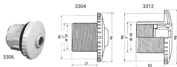
Boquilla de impulsión orientable 2" - 50 para encolar, para piscina Hormigón y Poliéster
