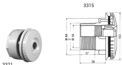
Boquilla de impulsión orientable 2"- 50 para encolar, para piscina Liner y Paneles
