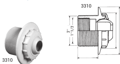
Boquilla de impulsión orientable 2" - 1 1/2" para piscina Hormigón
