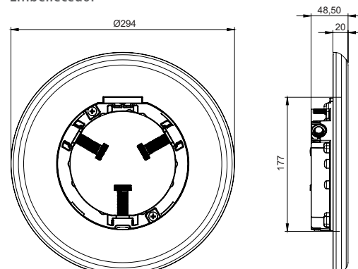
Embellecedor
